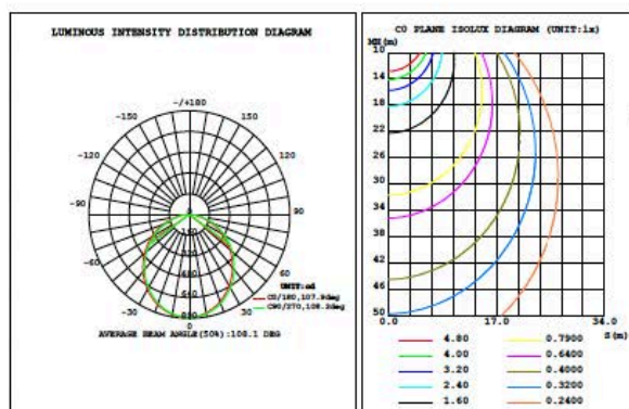
WSD-SDW101520W347-345K-W (20W&3000K)
