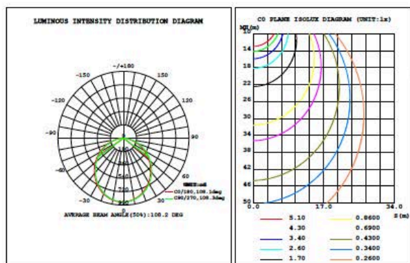
WSD-SDW101520W347-345K-W (20W&4000K)
