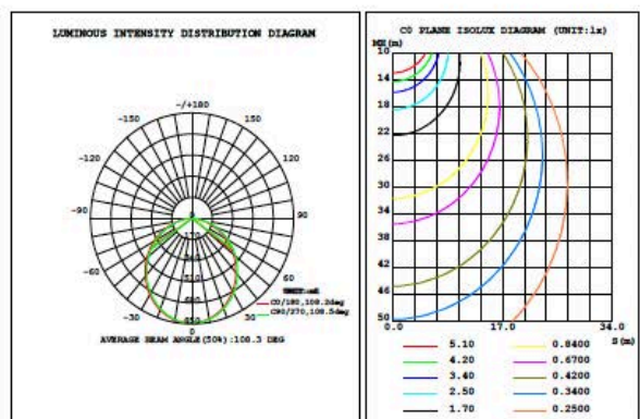
WSD-SDW101520W347-345K-W (20W&5000K)
